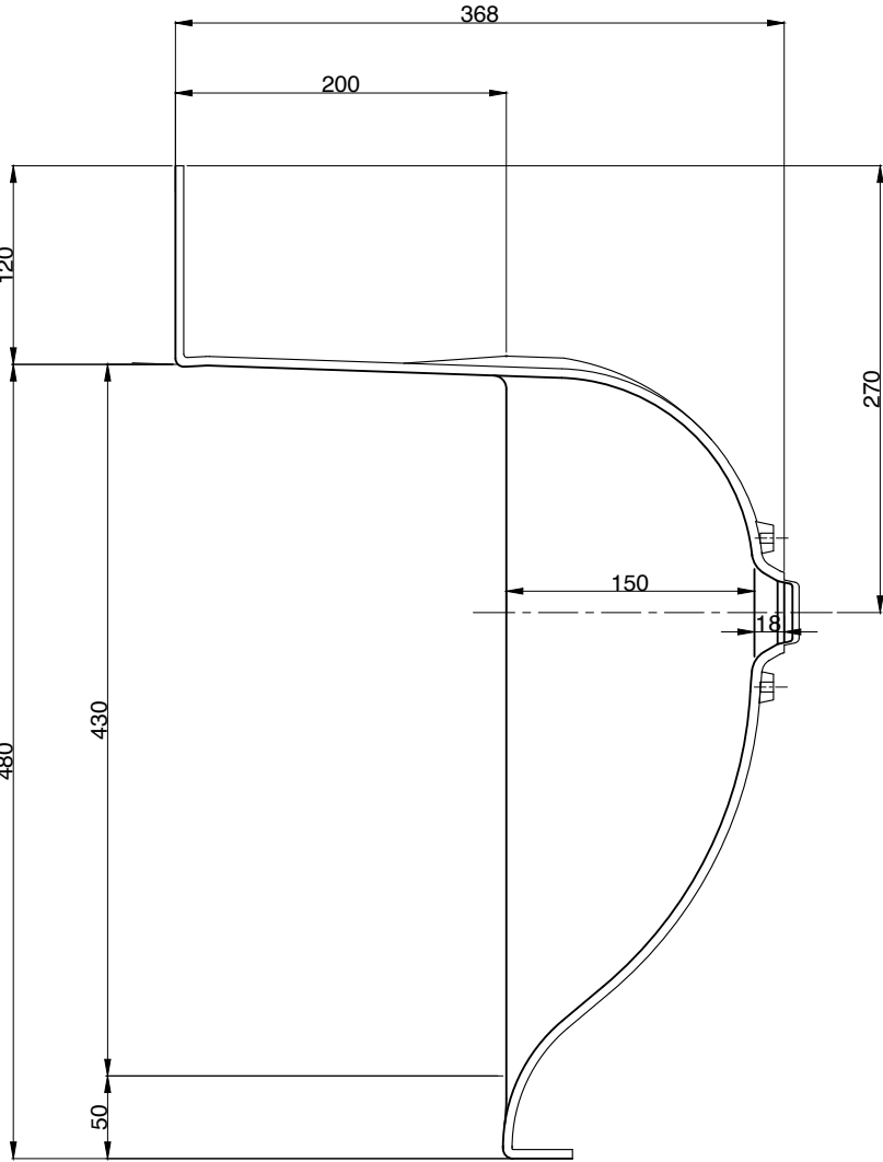
Section A-A
