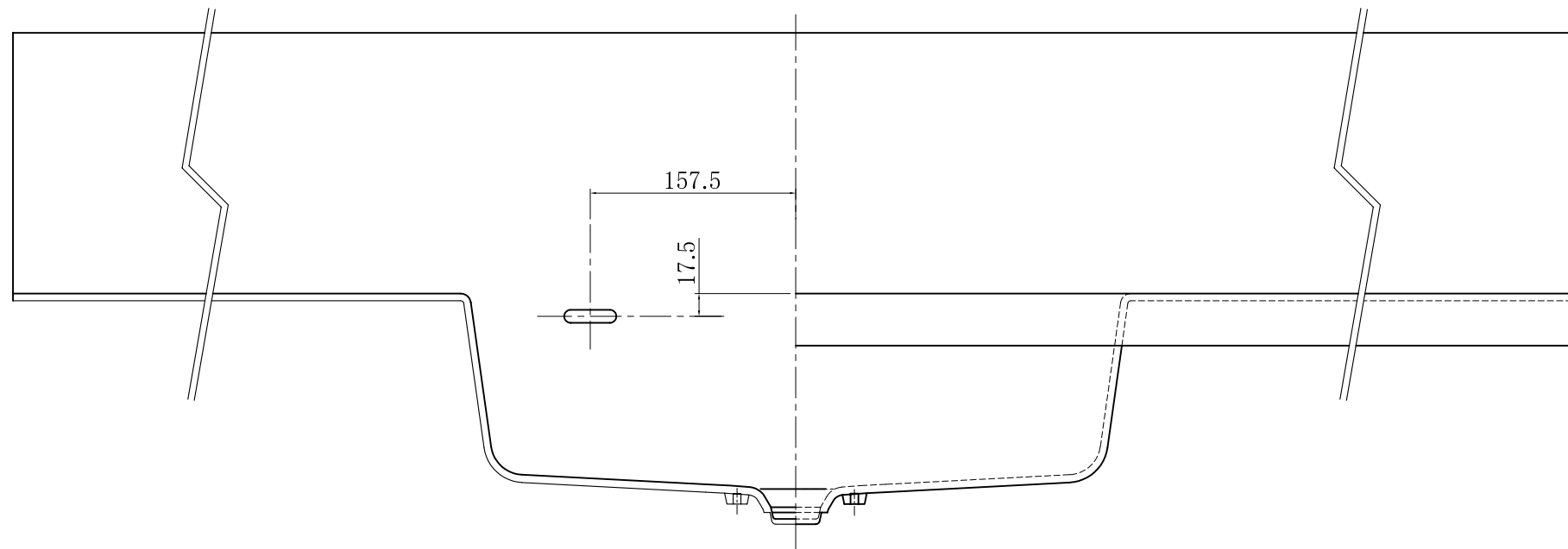
断面 B-B
