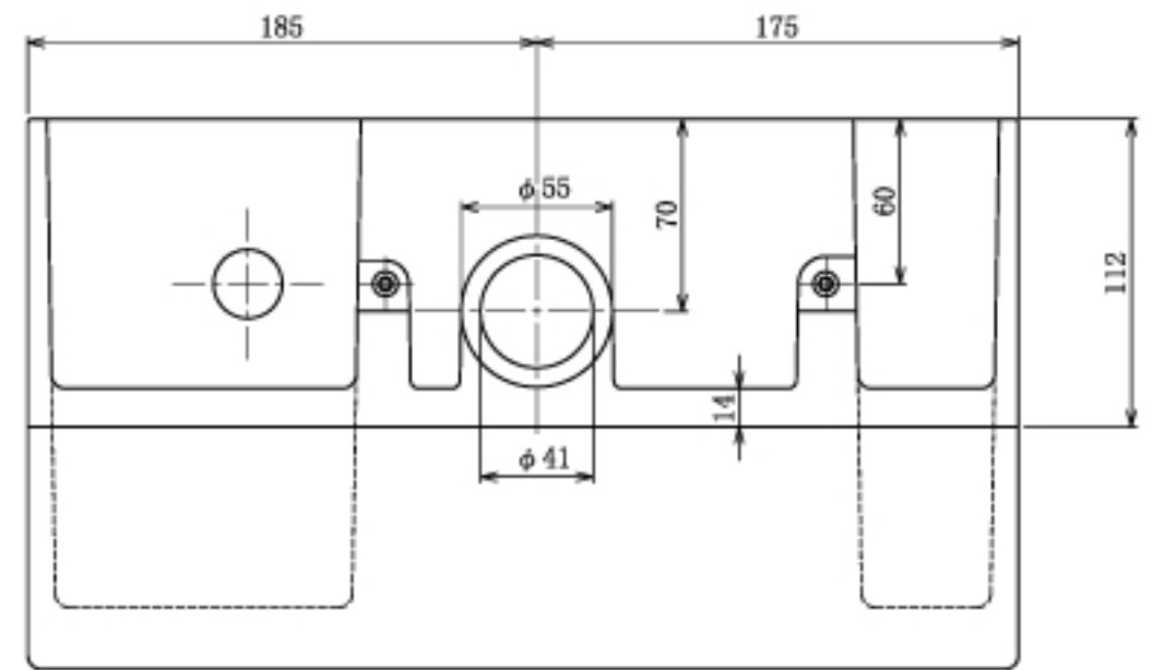
底面図
