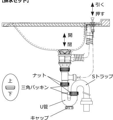
【排水セット】
