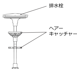
【弁セット】
